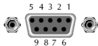
外部信号控制接口 插头引脚
